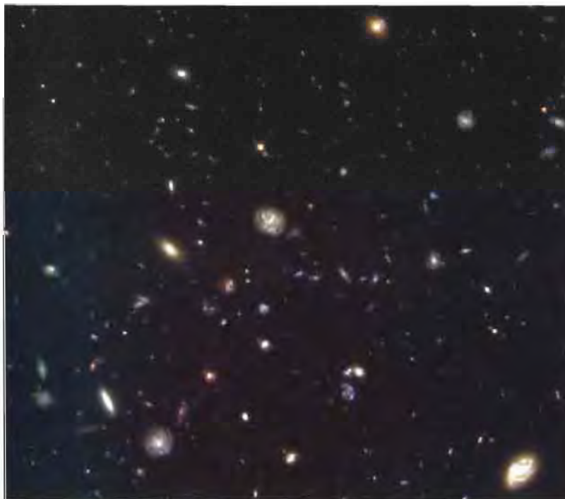
Илл. 5. Участок неба, который можно закрыть булавочной головкой, если ее держать на расстоянии вытянутой руки. При увеличении, как на этой иллюстрации, на данном участке открывается плотная область далеких галактик, каждая из которых содержит десятки миллиардов звезд. Фотография сделана космическим телескопом Хаббл во время десятидневного наблюдения над южным полушарием. (Фотография Р. Уильямса (STScI), HDF-S team, NASA)
