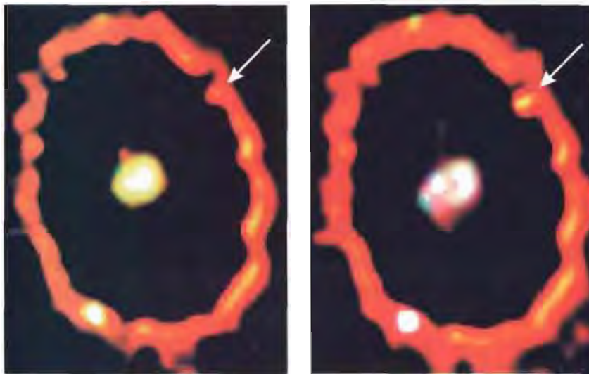
Илл. 4. Сверхновая SN1987A. Наблюдения телескопа Хаббл показывают наполняющийся ярким светом узел сверху на правой стороне кольца, окружающего остаток сверхновой. Это место мощного столкновения между движущейся наружу взрывной волной и самыми крайними с внутренней стороны фракциями околозвездного кольца. Столкновение нагревает газ и заставляет его светиться. (Фотография П. Гарнавича из Гарвард-Смитсоновского астрофизического центра и НАСА)
