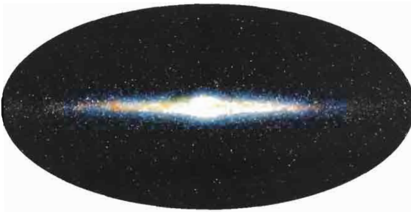
Илл. 2. Млечный путь в изображении спутника COBE (Cosmic Background Explorer). Фотография И.Л. Райта (UCLA). Проект COBE, DIRBE, NASA
