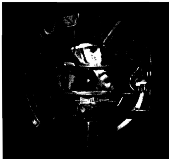
Рис. 12.1. На этой фотографии показано около миллиона атомов натрия, удерживаемых в магнитно-оптической ловушке, описанной в тексте. (С разрешения Национального института стандартов и технологии, Гейтерсбург, Мериленд.)
