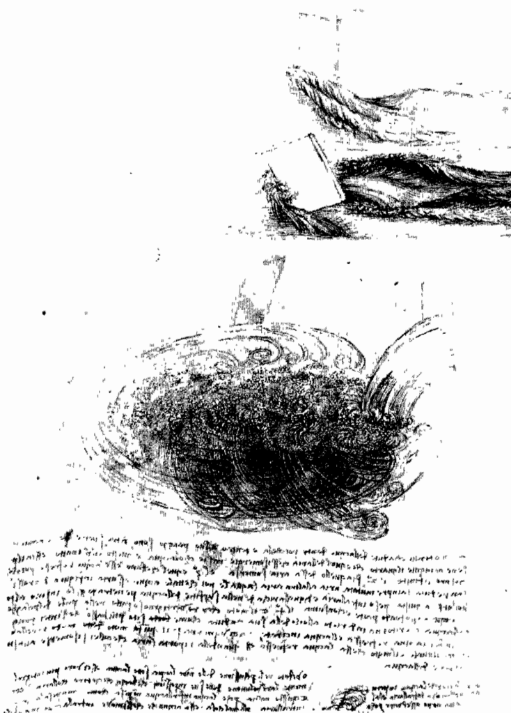
Рис. 5.1. Страница из записной тетради Леонардо да Винчи с рисунками омутов в текущей воде. («Вода». С. 1507-9 из Королевской коллекции ©2001, Ее величества королевы Елизаветы II)
