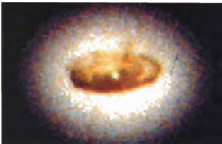
Илл. 17. Спиралевидный диск пыли питает массивную черную дыру в галактике NGC 4261. (Фотография Х.Форда и Д. Феррарезе (JHU), NASA)
