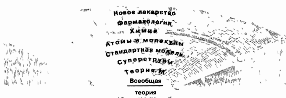
Рис. 1.2. Иерархия, связывающая основные законы природы с их практическим использованием. Необходимо проделать большой путь от всеобщей теории до получения нового лекарства
